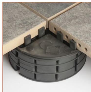
Maxi-Lager 20/4x10 (2fach) und Maxi-Lager 10/4x20 mit 2 Maxi-Ausgleichs-scheiben gestapelt und verlegt unter einer Keramikplatte
