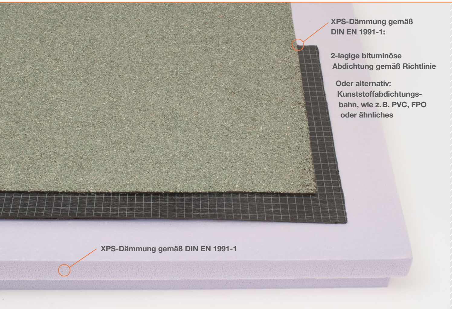
XPS-Wärmedämmung mit Abdichtungsbeispiel Bituminös
